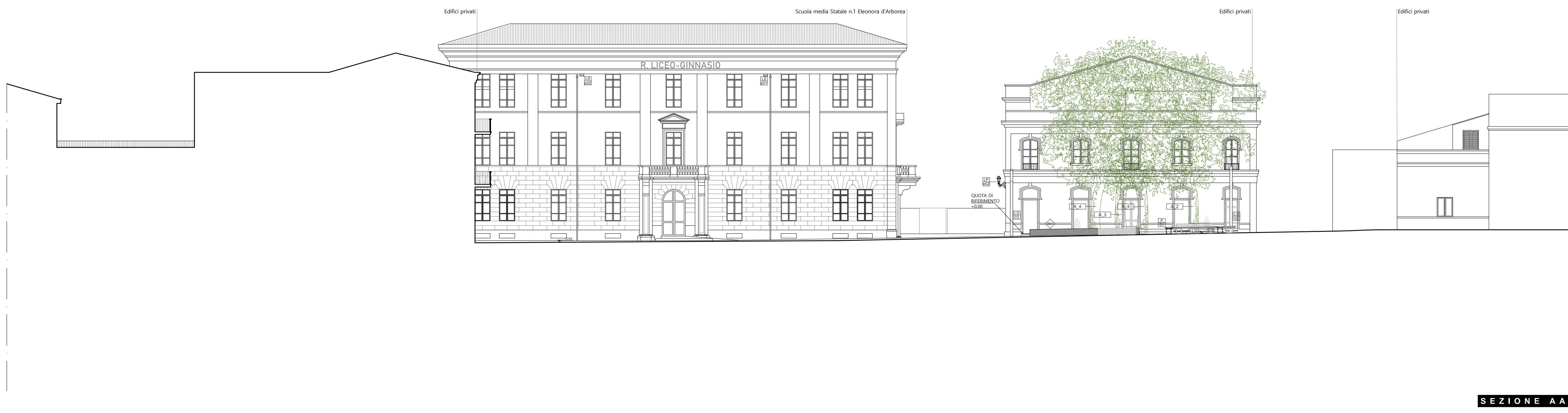
SEZIONE AA'
