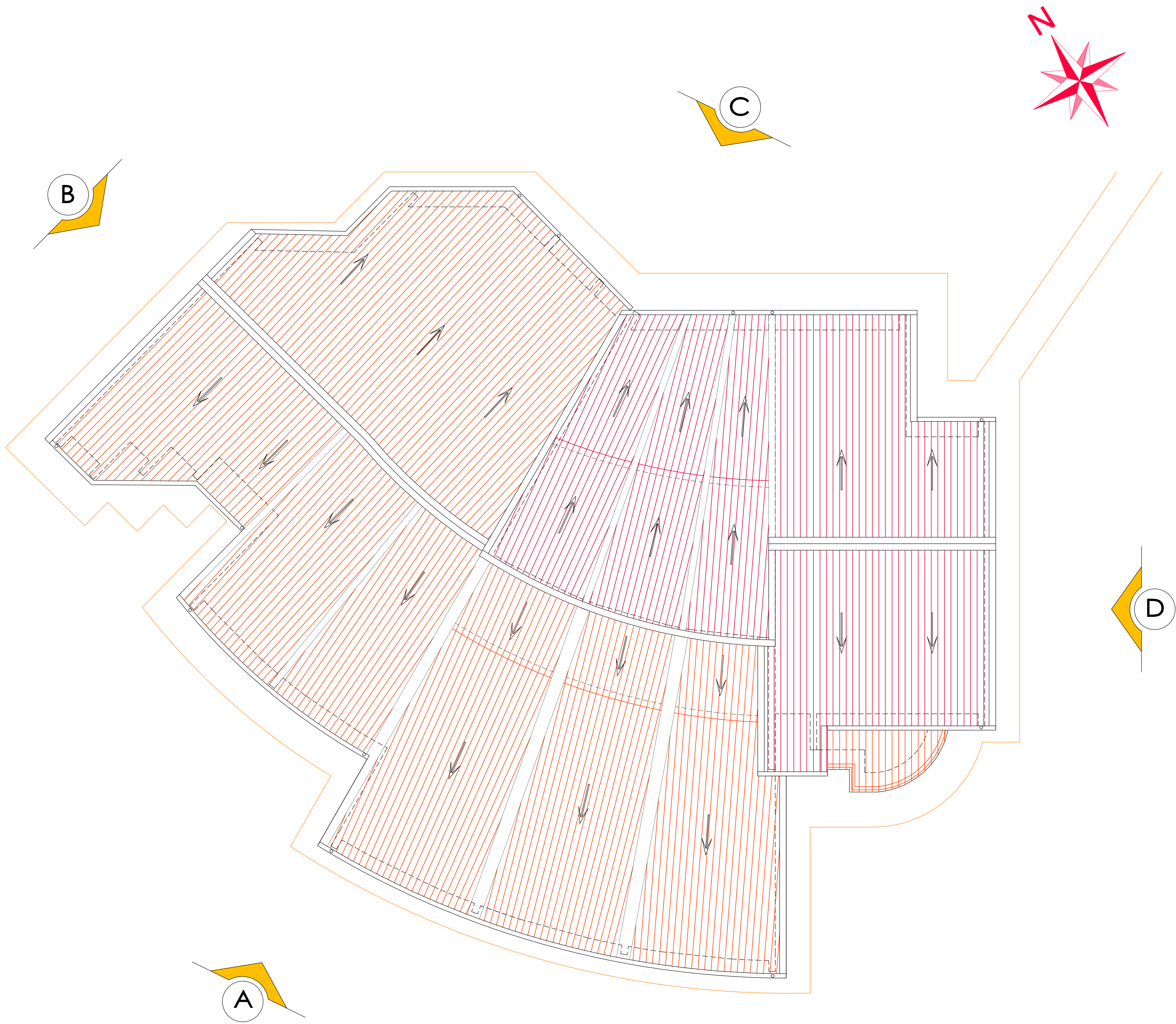
PIANTA COPERTURA - Scala 1:100
