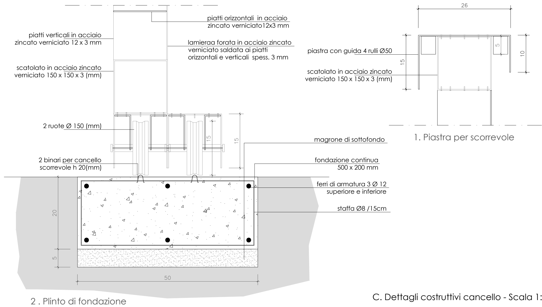
C. Dettagli costruttivi cancello - Scala 1:5
