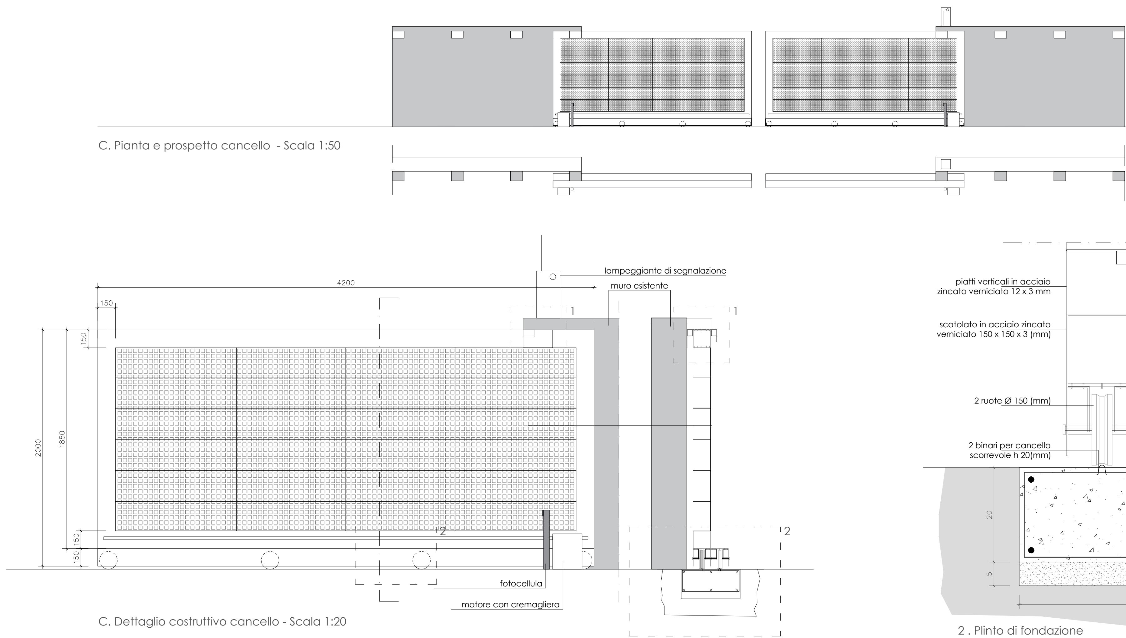
C. Dettaglio costruttivo cancello - Scala 1:20
