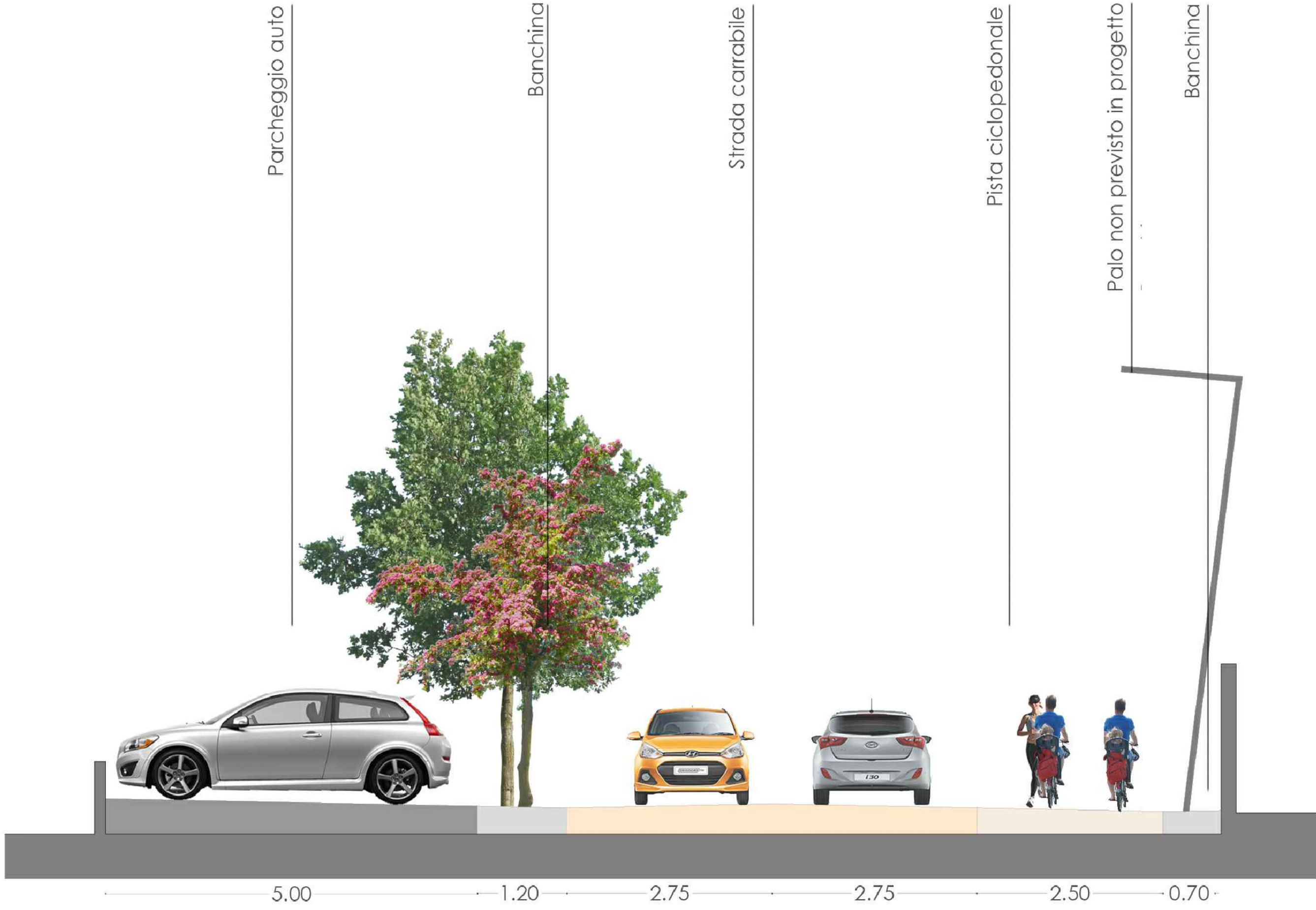
B. Sezione stradale - Scala 1:50
