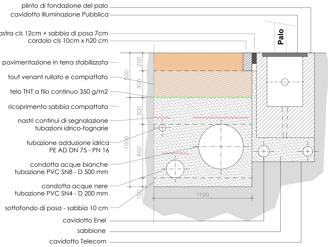
A. Particolare costruttivo - sezione sottoservizi Scala 1:20
