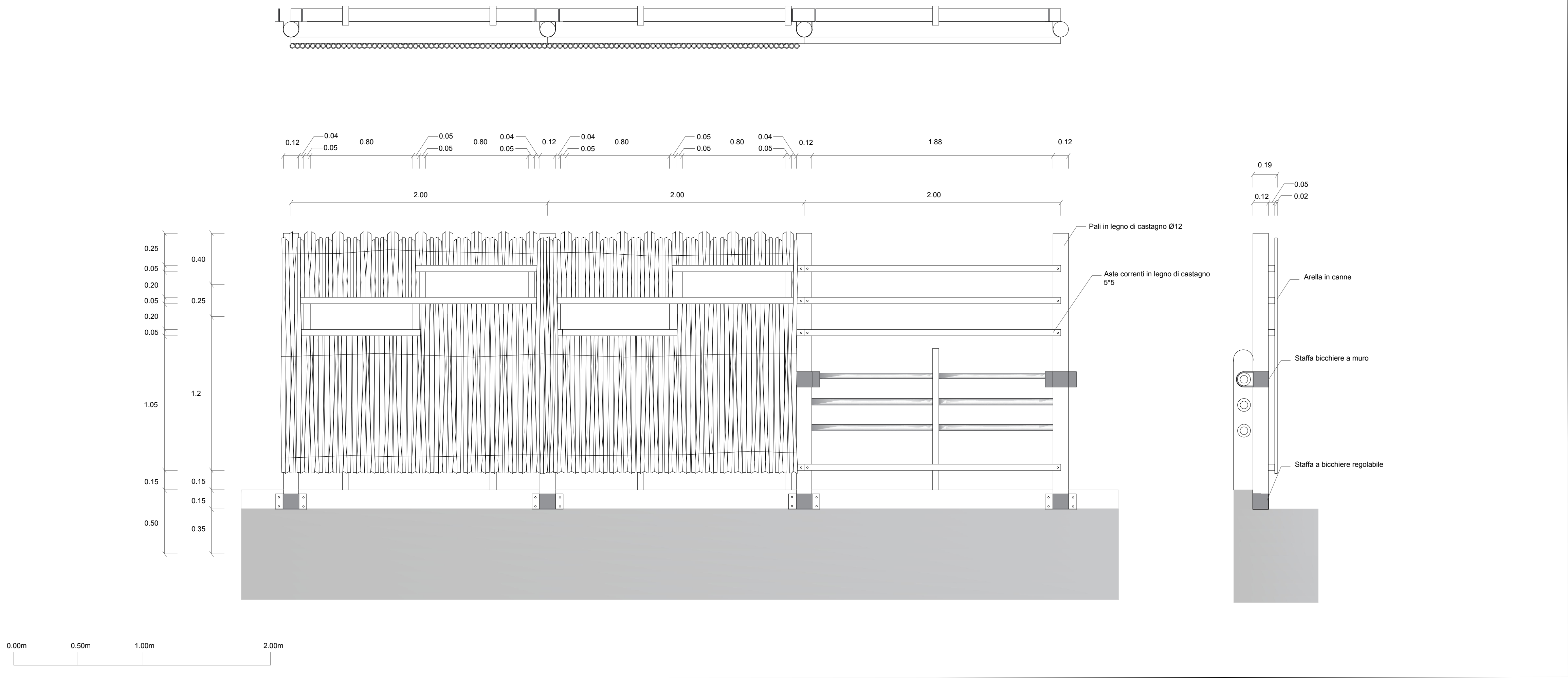
Particolare costruttivo: quinte in canna tipologia "c.1" scala 1:20
