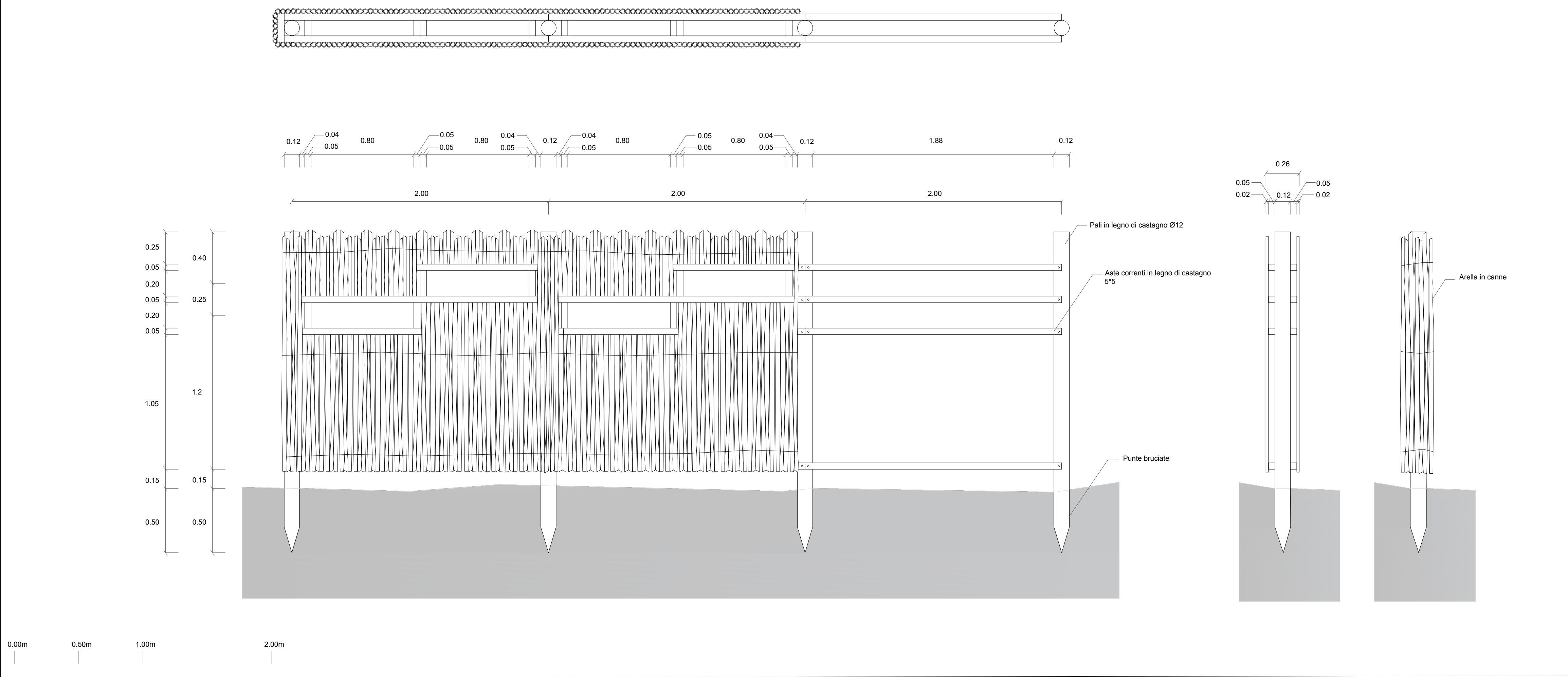
Particolare costruttivo: quinte in canna tipologia "c.2" scala 1:20
