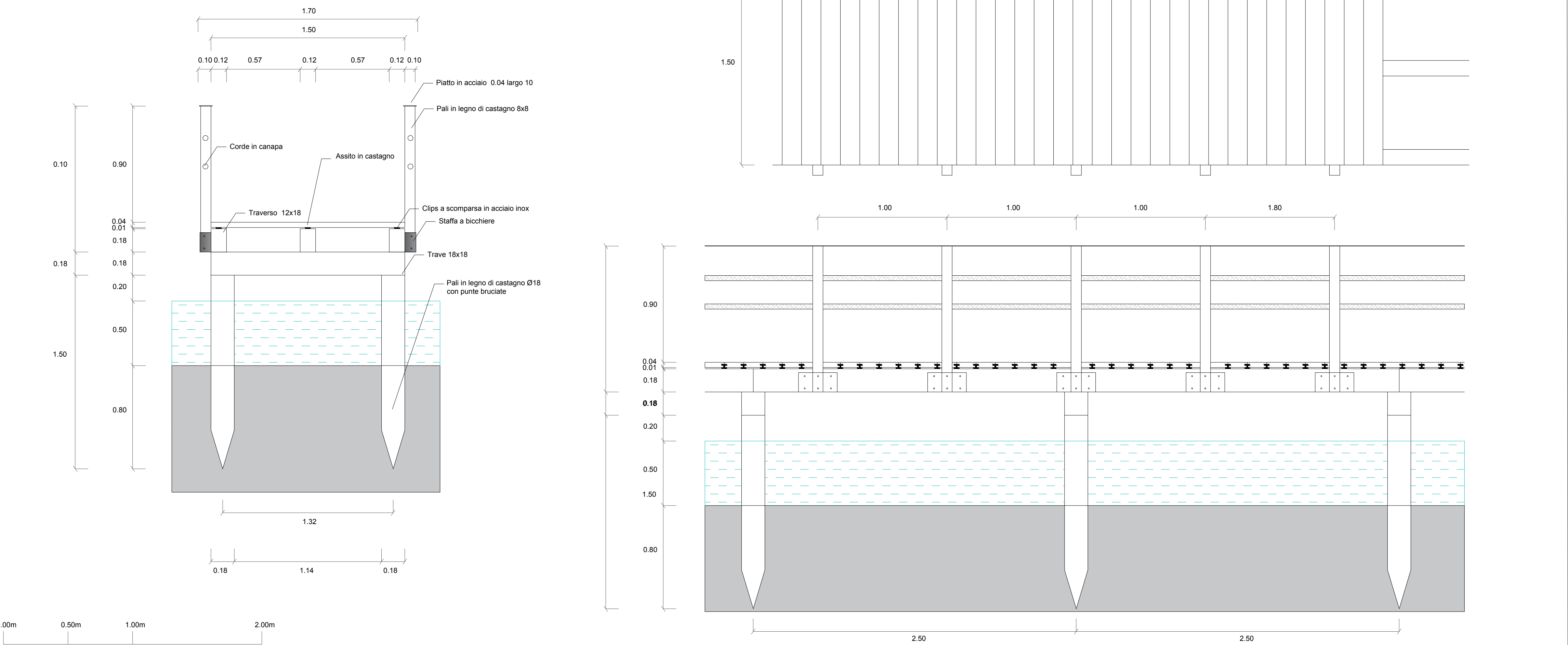
Particolare costruttivo: passerella tipologia "d.1" scala 1:20
