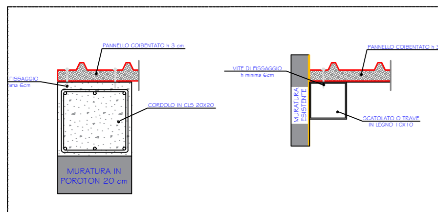
PARTICOLARE FISSAGGIO PANNELLO COIBENTATO 3cm SU CORDOLO E SCATOLATO
