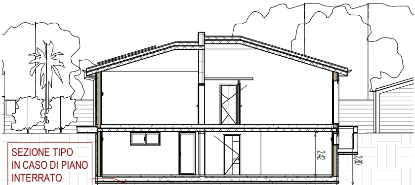
SEZIONE TIPO - Tip.Ed. 1 scala 1:200
