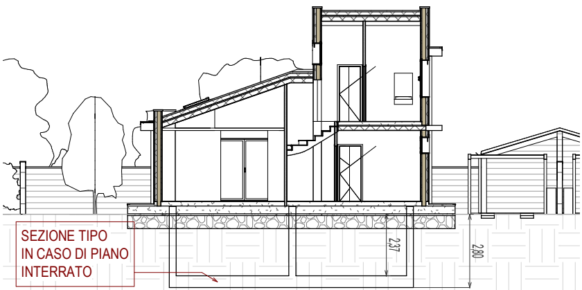
SEZIONE TIPO - Tip.Ed. 2 scala 1:200
