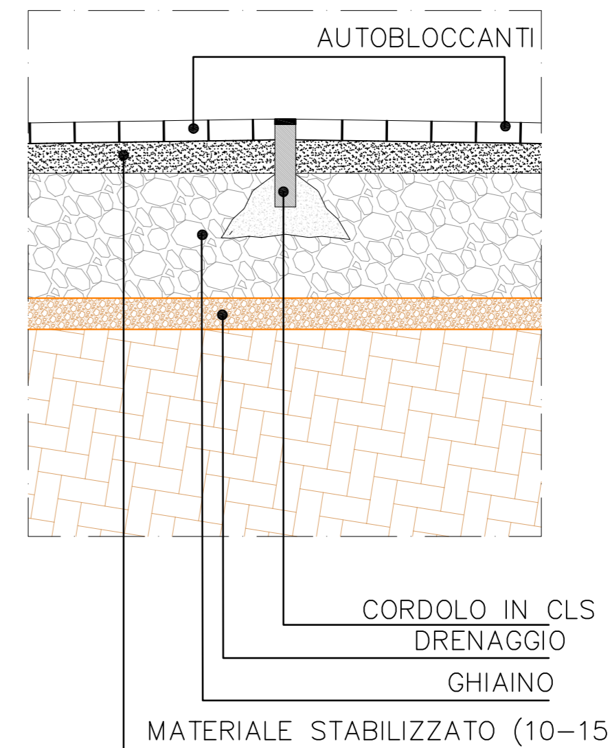
PARTICOLARE 4 SCALA 1:20
