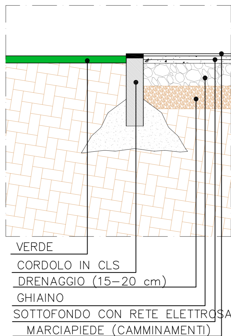
PARTICOLARE 1 SCALA 1:20
