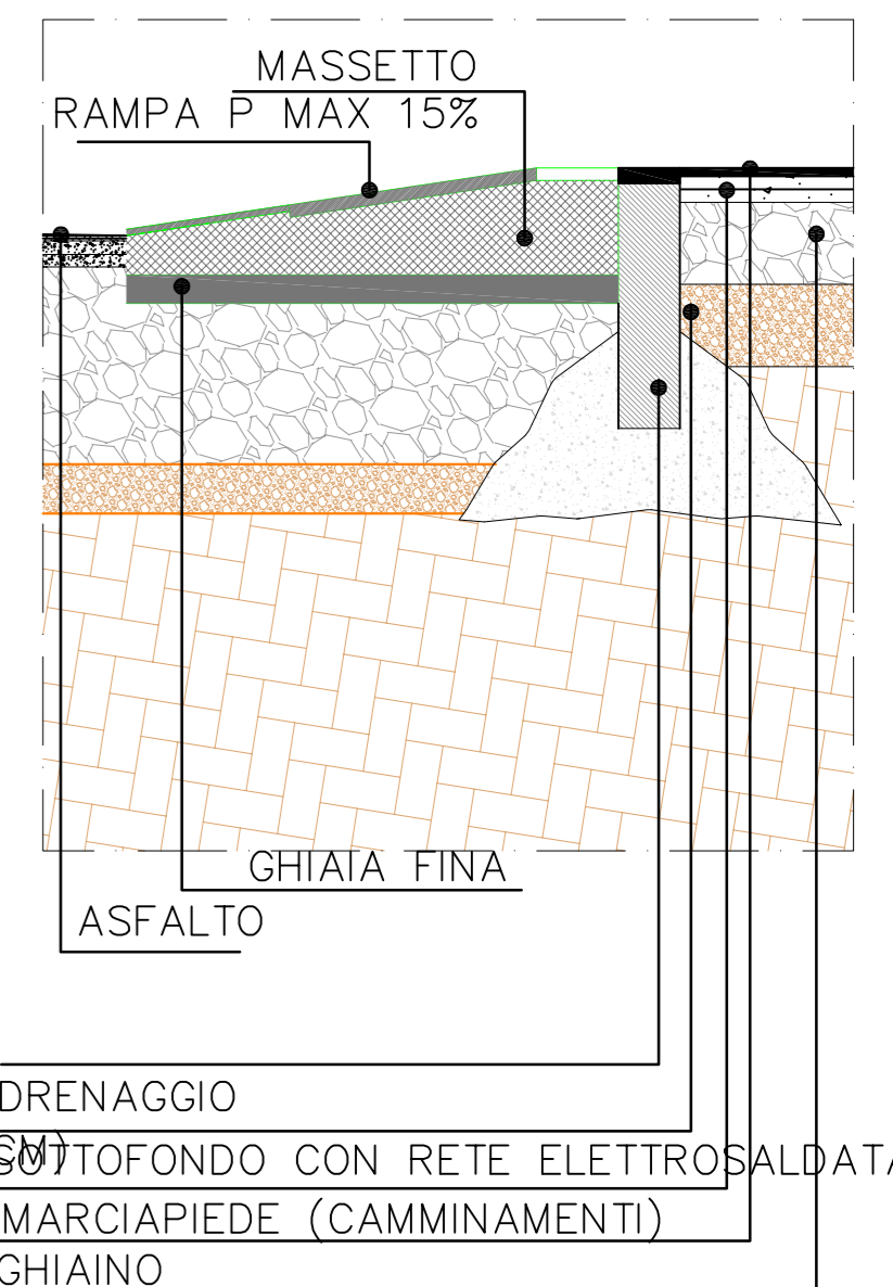
PARTICOLARE 5 SCALA 1:20
