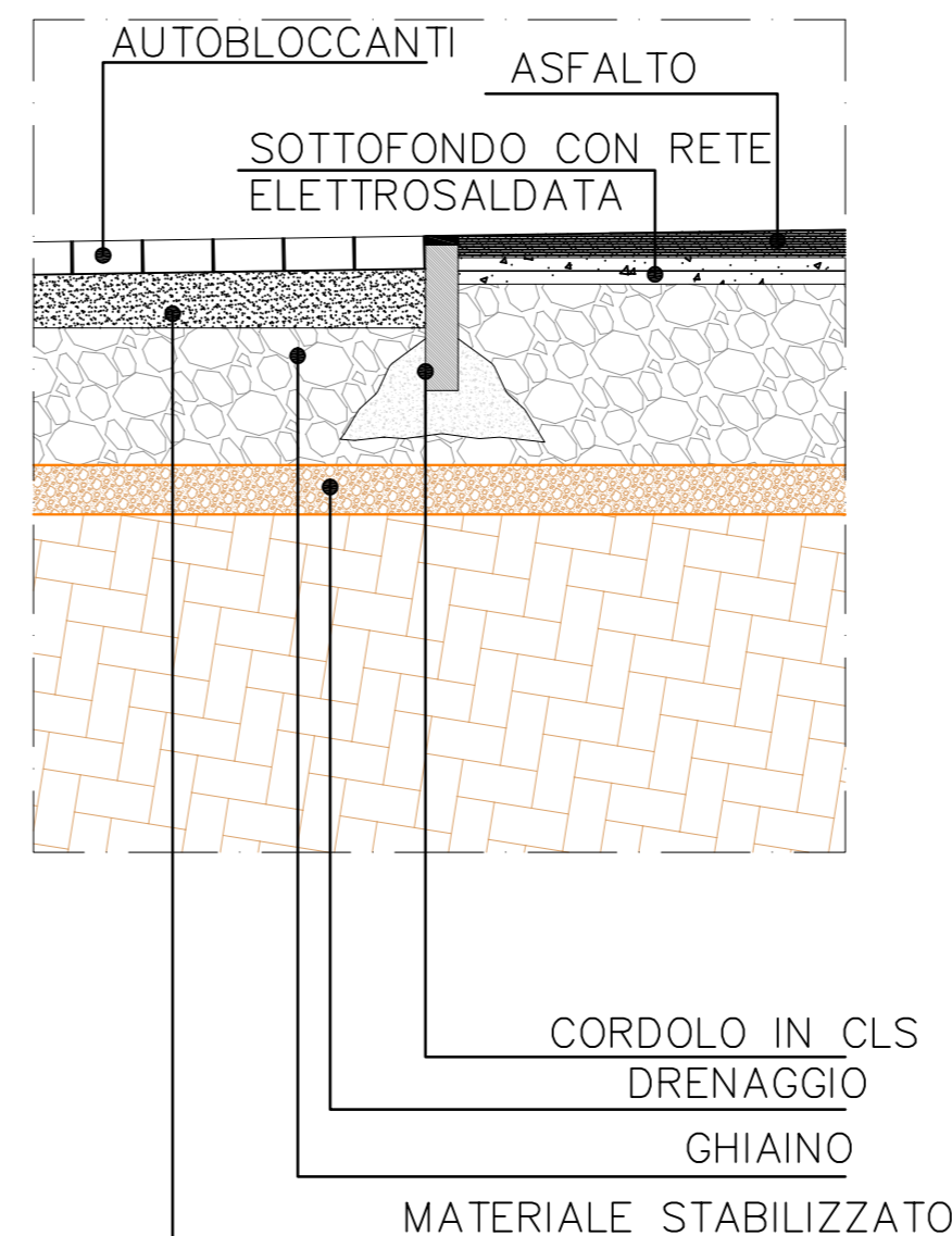
PARTICOLARE 3 SCALA 1:20
