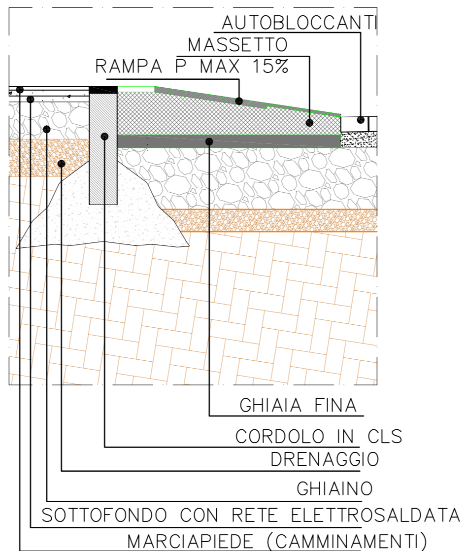
PARTICOLARE 2 SCALA 1:20
