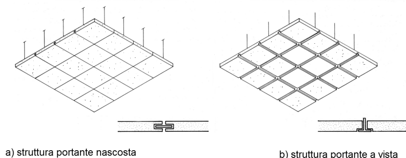
b) struttura portante a vista
