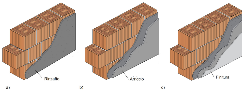
Stati componenti l'intonaco su una muratura di compannamento in laterizio
