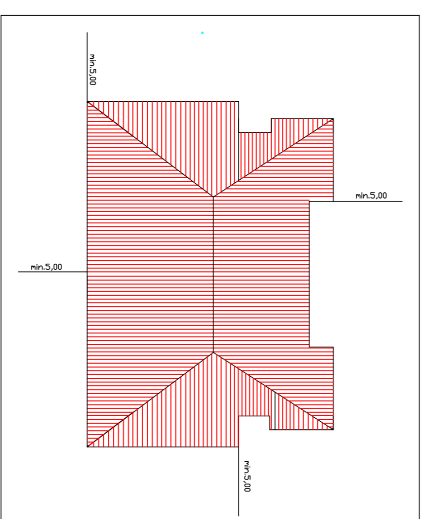
TIPOLOGIA SINGOLA o BINATA PIANTE COPERTIVE
