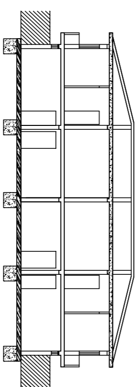
TIPOLOGIA SINGOLA o BINATA SEZIONE AA
